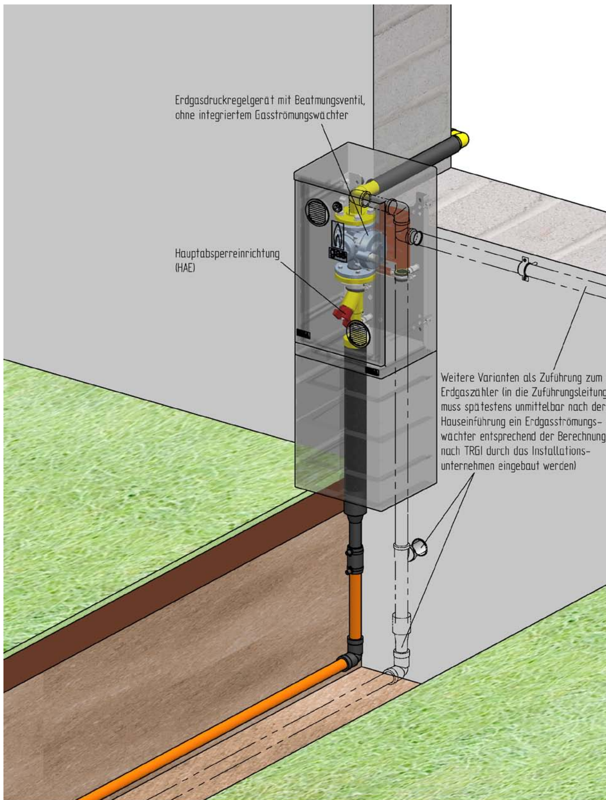
Die Befestigung des Kastens und der Hausanschlusskomponenten mit einer metallenen Montageplatten an der Außenwand kann bei fachgerechter Montage als ausreichende Ausziehsicherung für alle Einführungsvarianten im Sinne des Arbeitsblattes G459/I angesehen werden.
